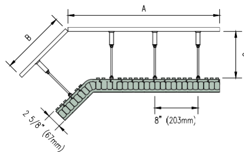
Серия One - Външен 45° Ъгъл One Side Outside 45° Corner
