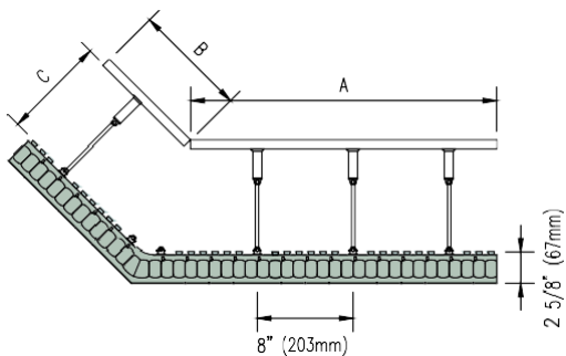
Серия One - Вътрешен 45° Ъгъл
