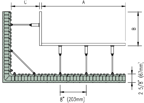
Серия One - Вътрешен Ъгъл 90° Corner
